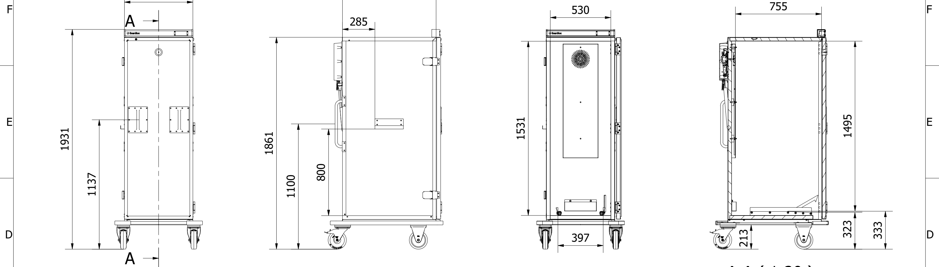
A-A ( 1:20 )
