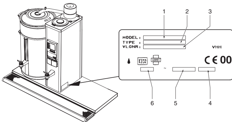
Fig. 1 ID-plate
