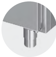
Adjustable heavy duty stainless steel feet (amplitude 60 mm +10/-50) Pieds réglables robustes en inox (amplitude de 60 mm +10/-50 mm) Höhenverstellbare Schwerlastfüße aus Edelstahl (Umfang: 60 mm +10/-50)
